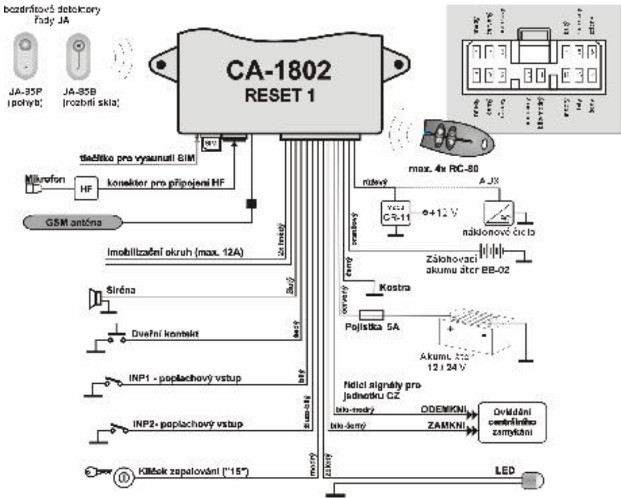
Obr. 1: Zapojení alarmu v profilu RESET 1. V tomto zapojení je autoalarm schopen ovládat centrální zamykání vozu.
